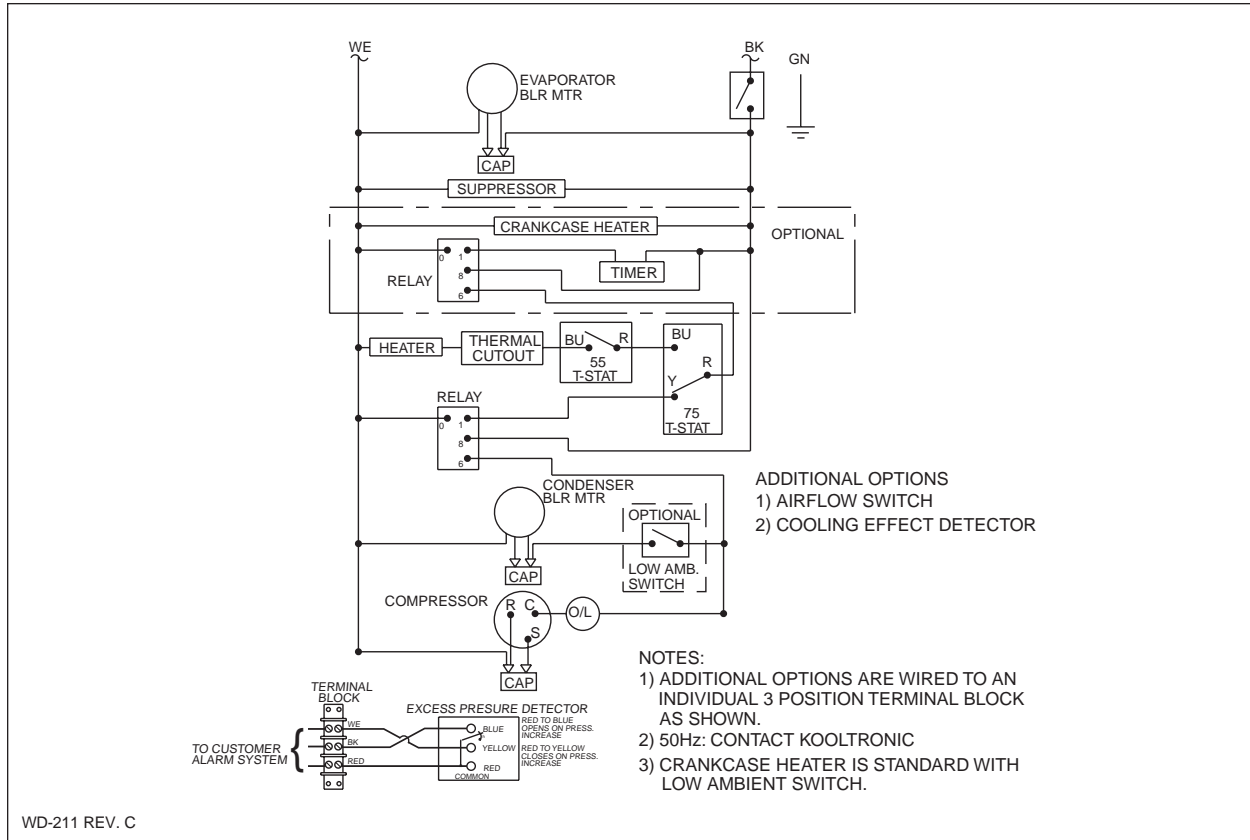
WD-211 REV. C
