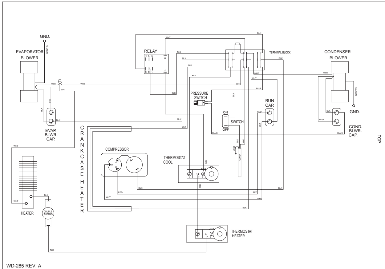
WD-285 REV. A
